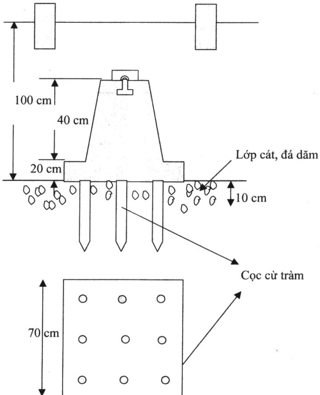
Hình 5. Mốc thường vùng đất yếu
