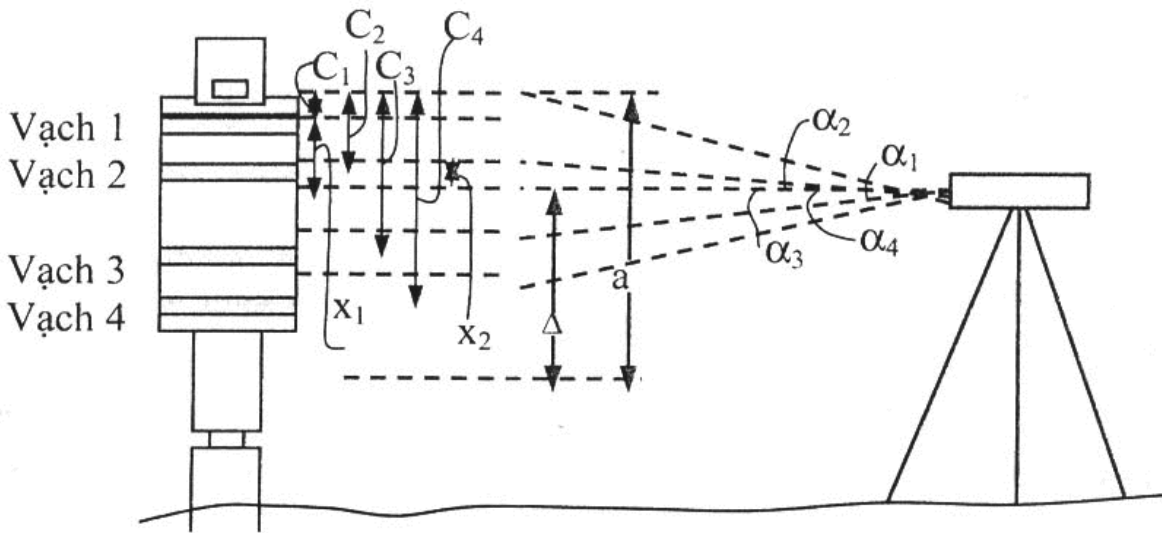
Hình vẽ đo qua sông bằng phương pháp tia ngắm nghiêng
