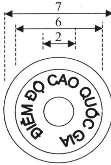
Hình 8. Dấu kim loại
