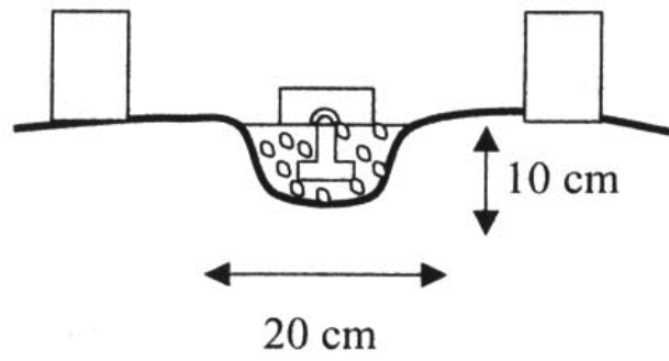
Hình 5. Mốc thường vùng đất yếu
