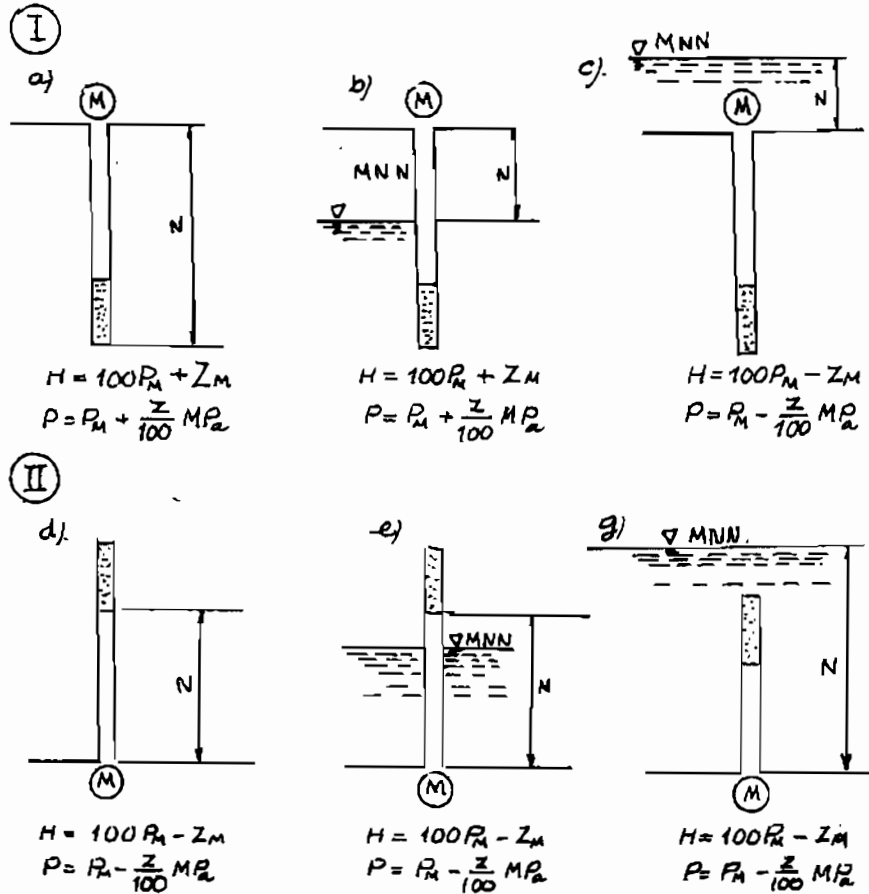
Hình 1 - Tính áp lực tác động trong đoạn lỗ khoan khi thí nghiệm ép nước
