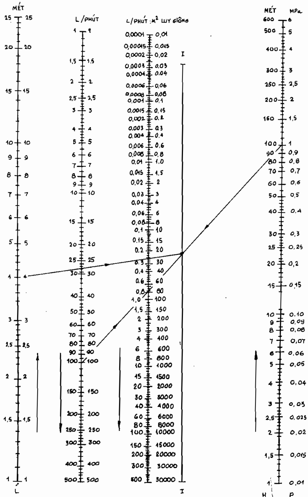
Hình 2.- Toán đồ để xác định lượng mất nước đơn vị ( q và \mu )
