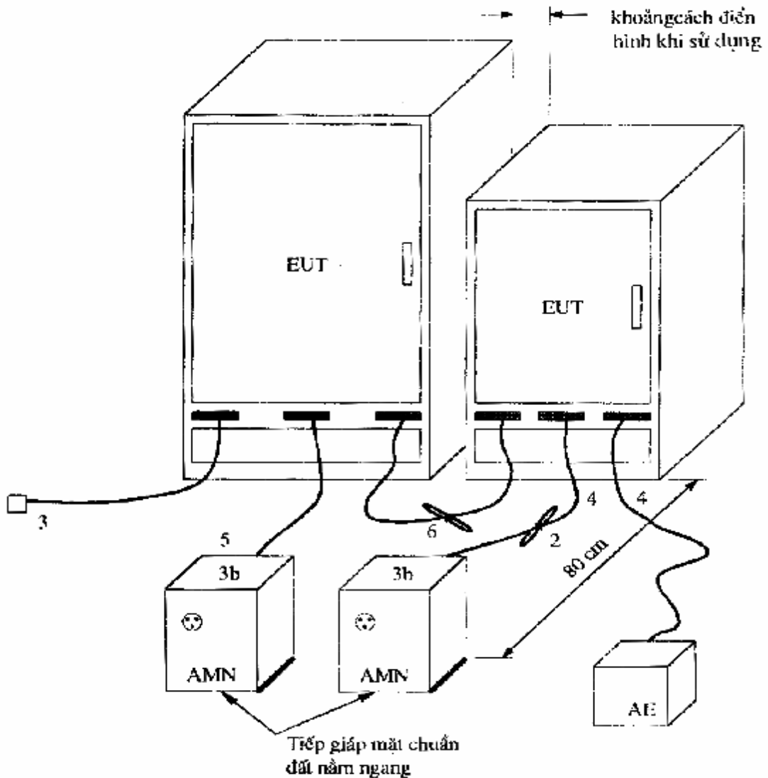
Hình 8: Cấu hình phép đo nhiễu dẫn cho các thiết bị đặt trên sàn nhà
