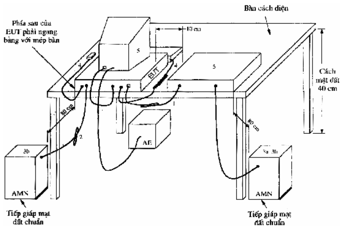
Hình 7: Cấu hình phép cho các thiết bị đặt bàn (Phép đo nhiễu dẫn tại một vị trí đo nhiễu phát xạ)
