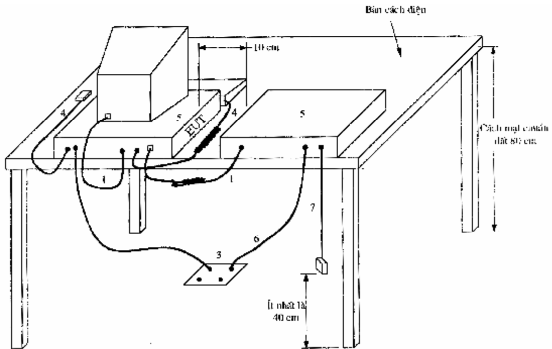
Hình 10: Cấu hình phép đo nhiễu phát xạ cho thiết bị đặt bàn
