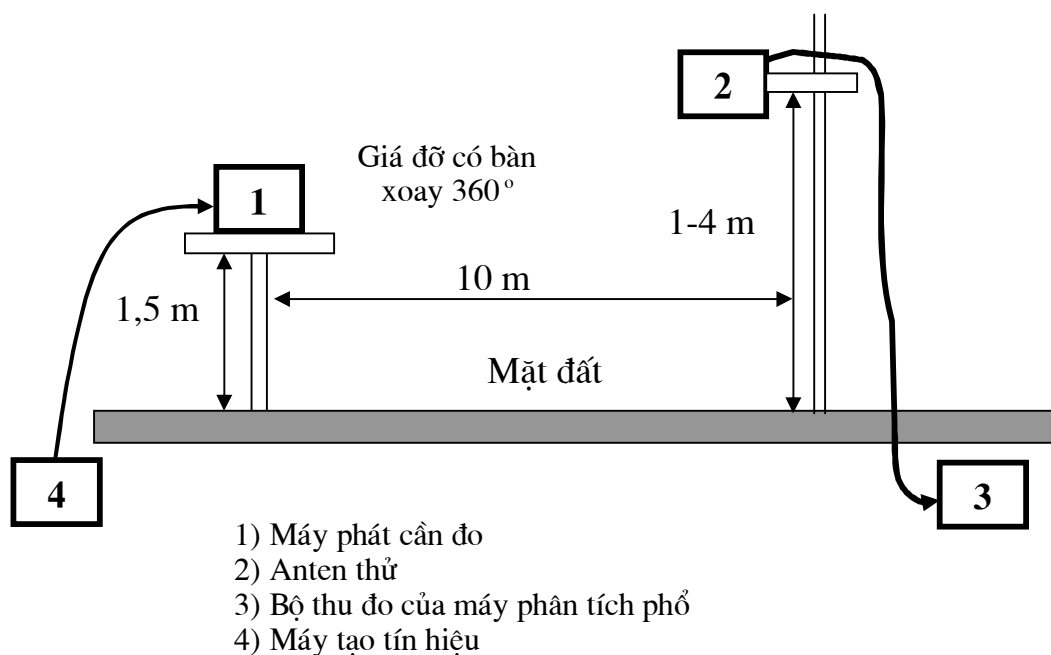
Hình 5: Sơ đồ đo công suất sóng mang gián tiếp
