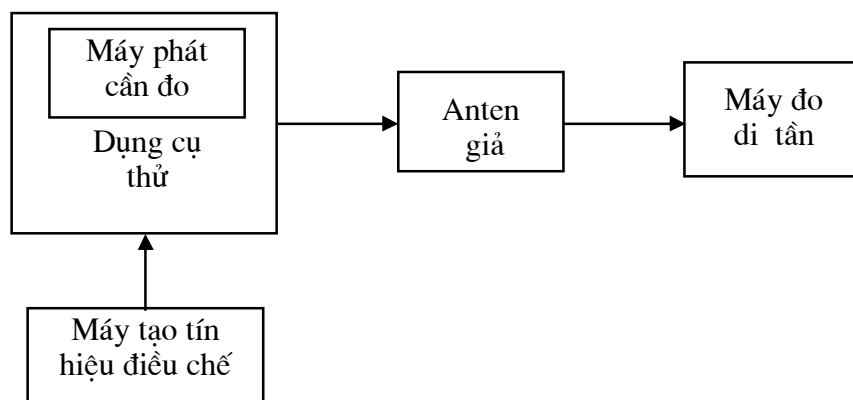
Hình 7: Sơ đồ đo độ di tần gián tiếp
