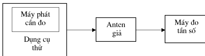
Hình 2: Sơ đồ bố trí đo tần số gián tiếp
