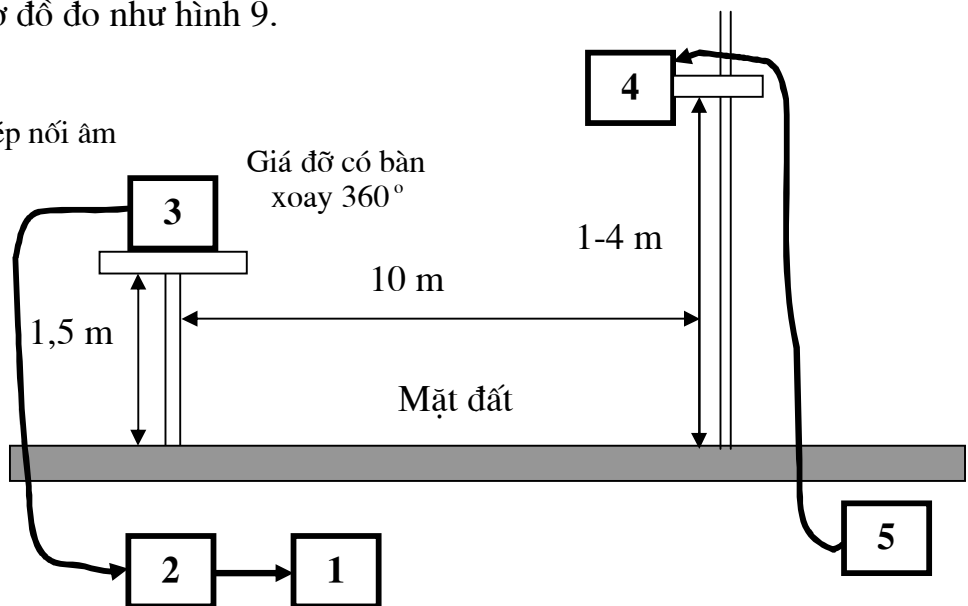
Hình 9: Sơ đồ đo độ nhạy gián tiếp của máy thu
