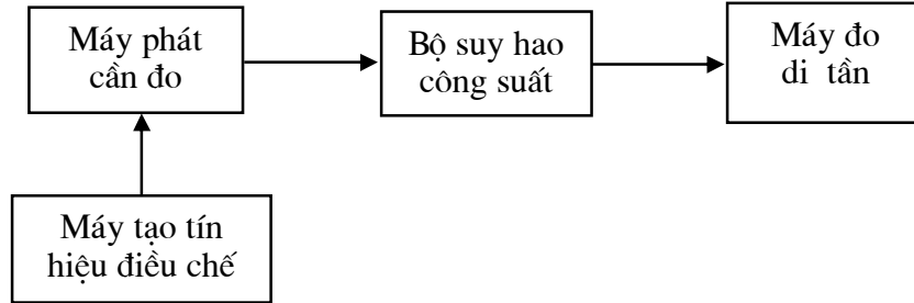
Hình 8: Sơ đồ đo độ di tần trực tiếp
