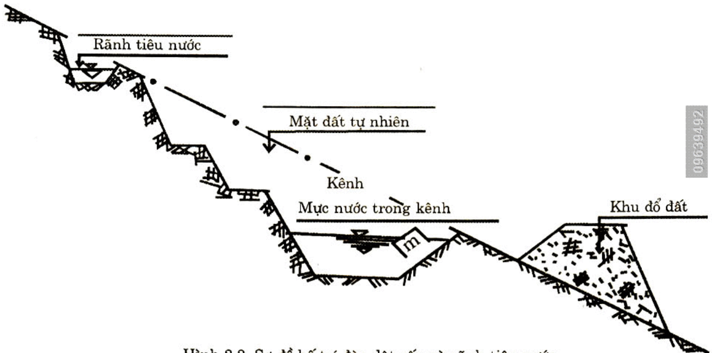
Hình 2.2. Sơ đồ bố trí đào dật cấp và rãnh tiêu nước
