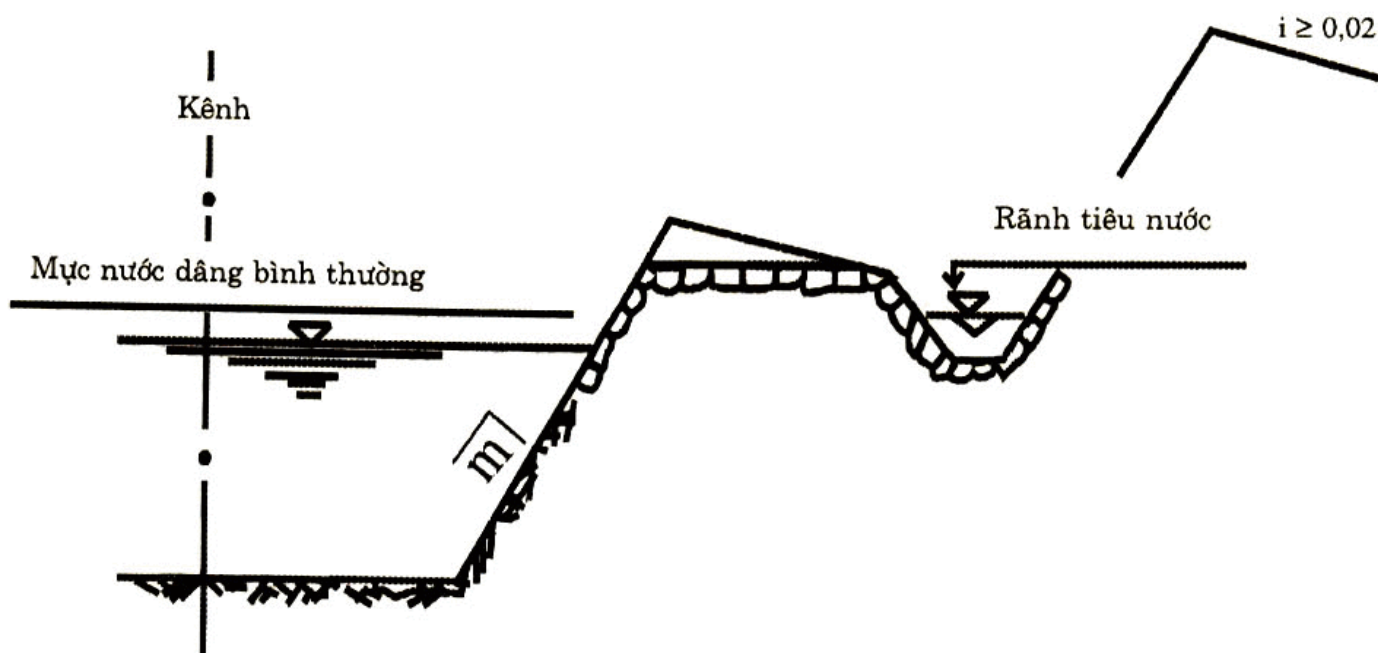
Hình 2.1. Sơ đồ bố trí đào và làm bờ kênh
