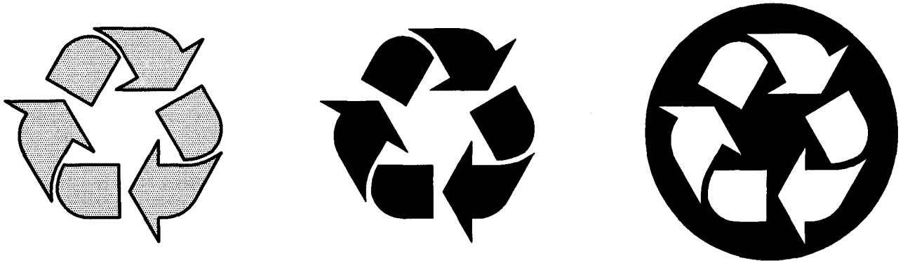
Hình 1 - Ví dụ về vòng Mobius
