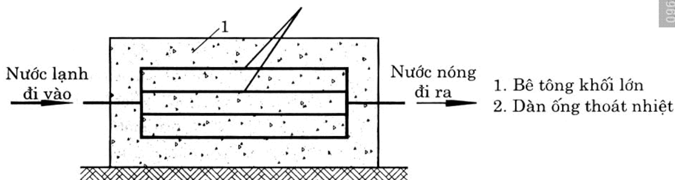
Hình 1. Sơ đồ đặt dàn ống thoát nhiệt cho khối lớn bê tông
