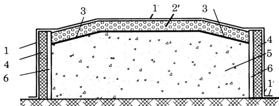
Hình 2. Sơ đồ bóc vật liệu cách nhiệt để giữ nhiệt khối đổ
