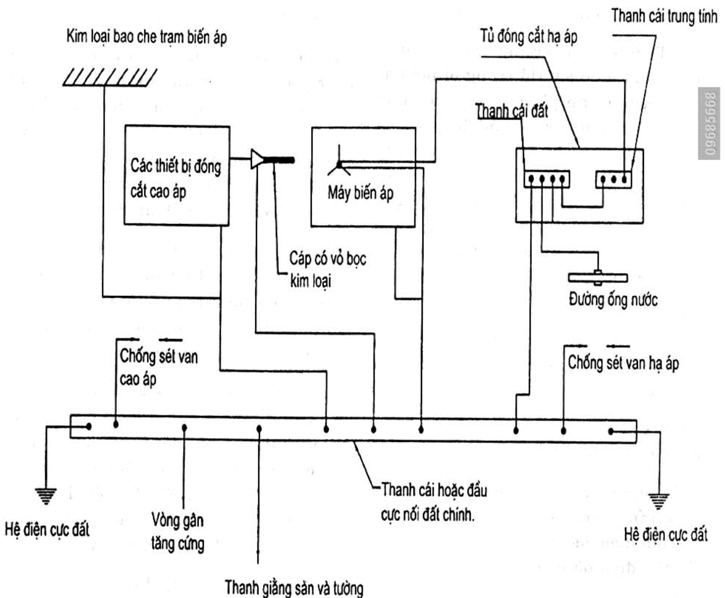
Hình 2. Hướng dẫn áp dụng hệ thống nối đất chung
