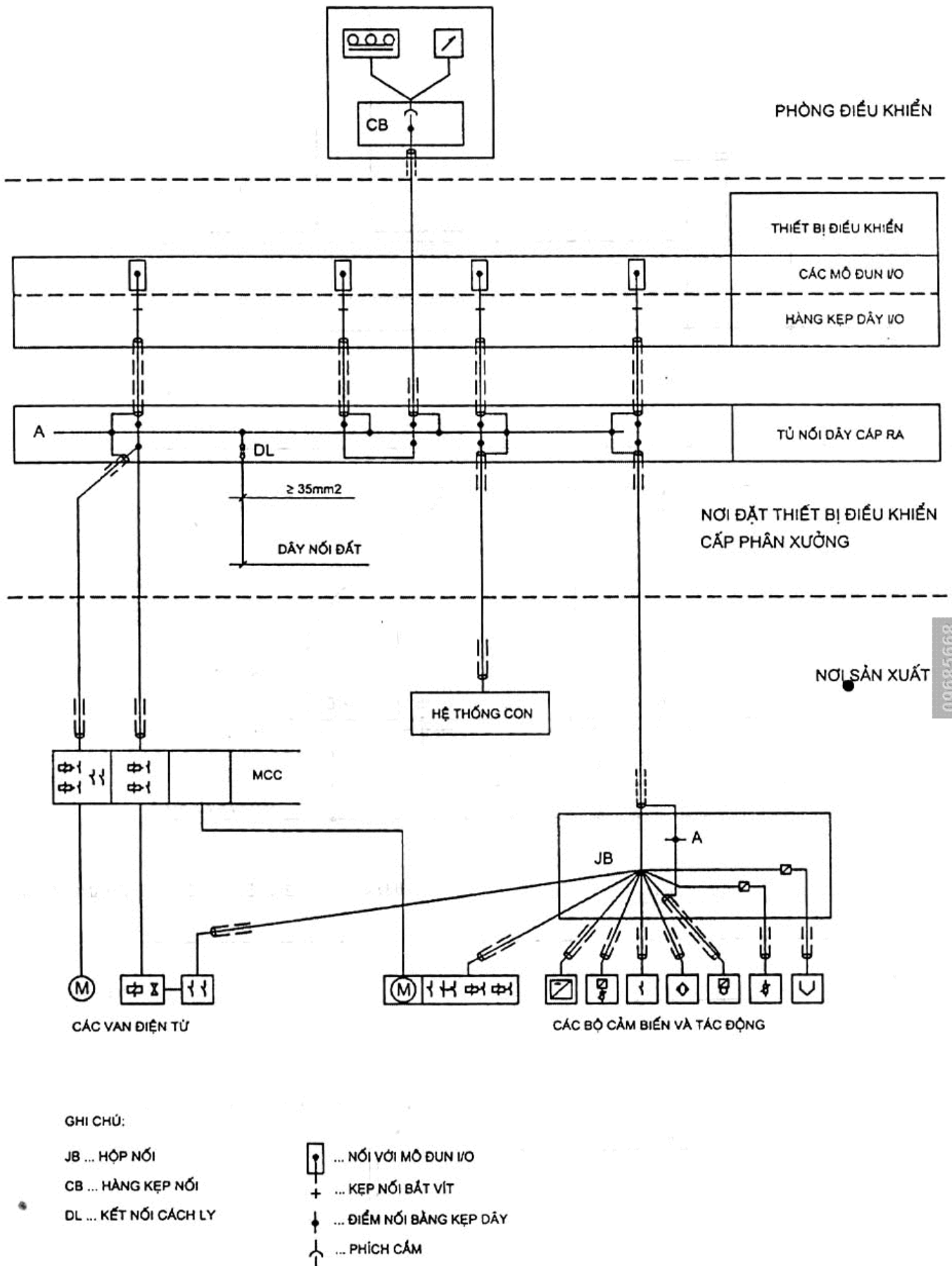
Hình 13: Nối đất chống nhiễu cho hệ thống điều khiển và giám sát sử dụng máy tính
