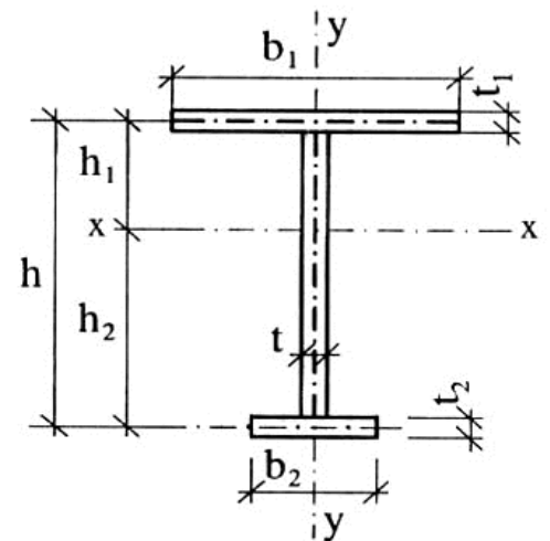
Hình E.1. Sơ đồ dầm tiết diện chữ I có một trục đối xứng
