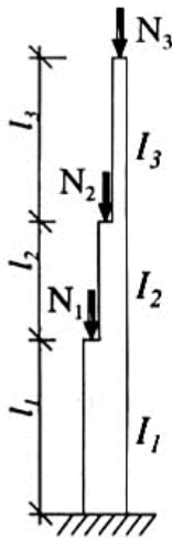
Hình D.2. Sơ đồ cột
