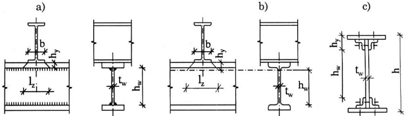
Hình 2 - Sơ đồ tính chiều dài phân bố tải trọng lên bụng dầm
