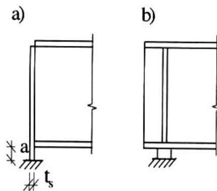
Hình 12 - Sơ đồ đặt sườn cứng ở gối
