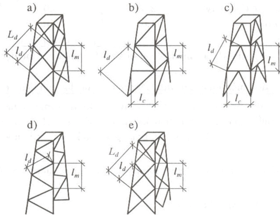
Hình 9 - Sơ đồ kết cấu không gian rộng, các thanh từ thép góc đơn
