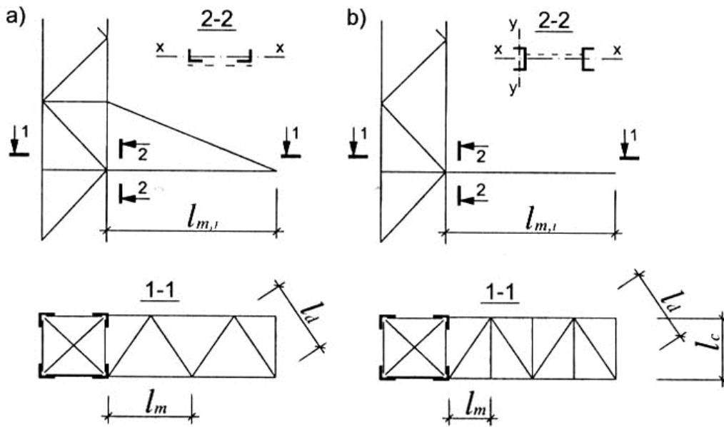
Hình 21. Sơ đồ xà ngang
