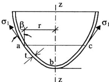
Hình 15 - Sơ đồ vỏ tròn xoay
