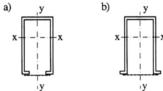
Hình 3 - Các cấu kiện có tiết diện dạng Π
