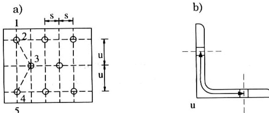
Hình 1 - Cách xác định diện tích thực
