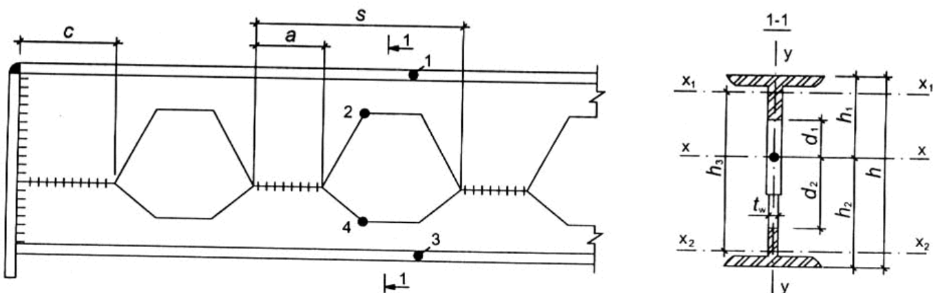
Hình 20. Sơ đồ một đoạn dầm có lỗ
