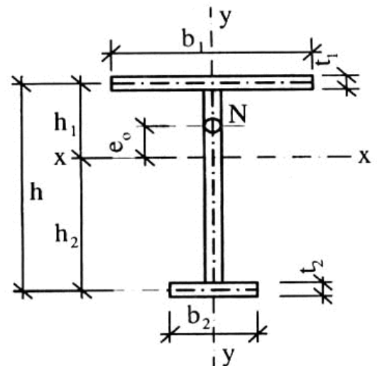
Hình D.4. Sơ đồ tiết diện chữ I một trục đối xứng chịu nén lệch tâm
