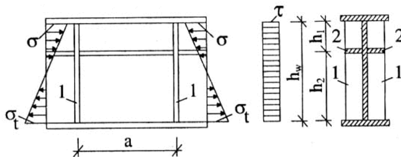
Hình 11 - Sơ đồ dầm được tăng cường bằng các sườn cứng dọc và ngang
