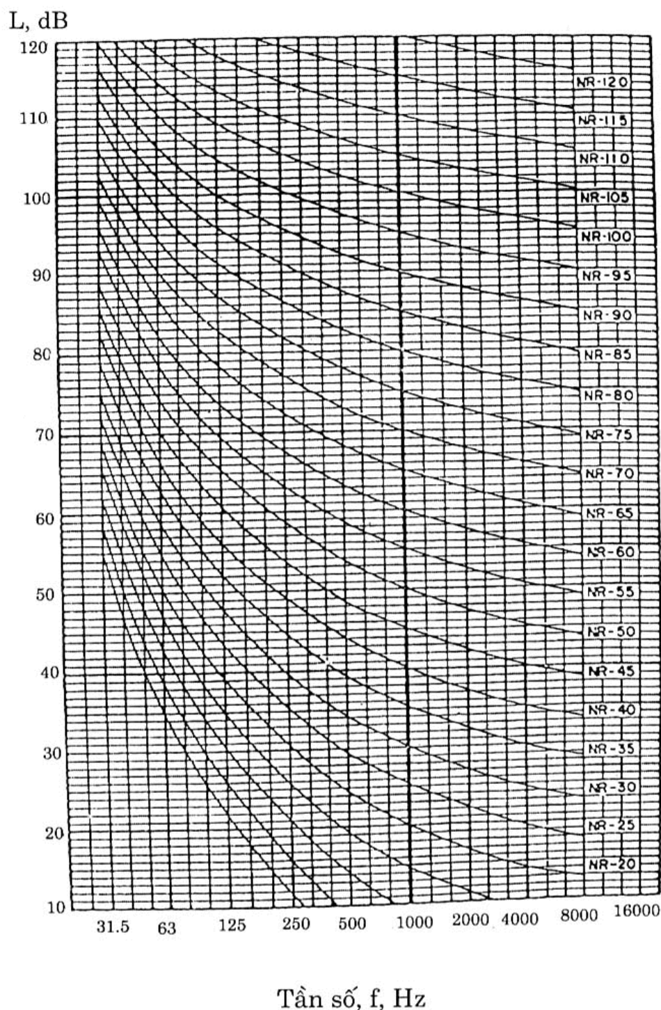
Hình 1. Họ đường cong NR (I.S.O. R 1996, 1971)
