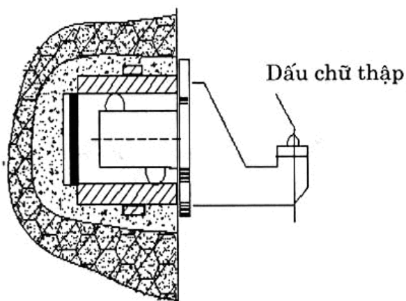
Hình B.1. Cấu tạo loại mố gắn vào công trình
