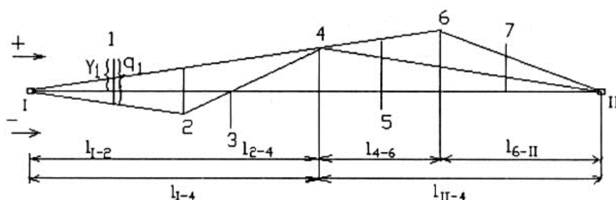
Hình D.2. Sơ đồ đo hướng chuẩn từng phần
