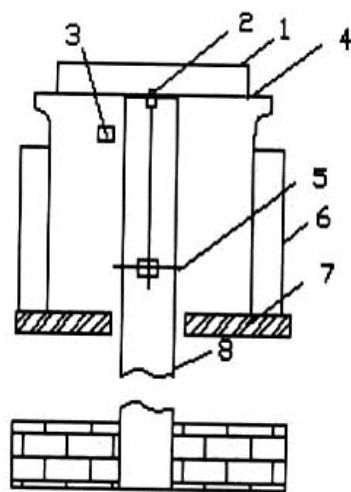
Hình A.1. Cấu tạo loại mố nổi
