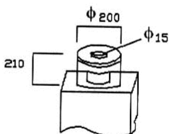
Hình A.2. Cấu tạo loại mố chìm
