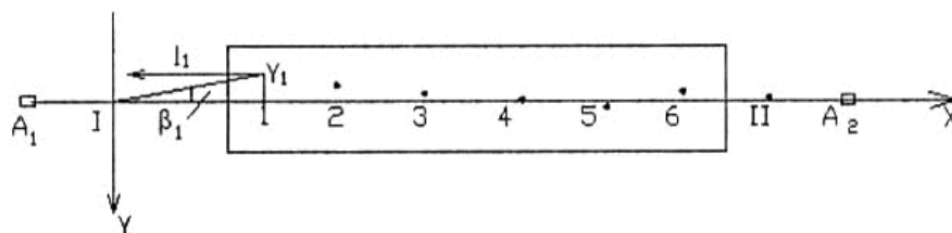
Hình 1. Sơ đồ vị trí mốc cơ sở và mốc kiểm tra chuyển dịch ngang
