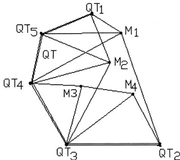
Hình F.1. Sơ đồ lưới quan trắc chuyển dịch ngang nhà máy thủy điện
