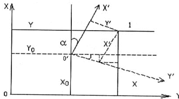
Hình 5. Sơ đồ biến đổi tọa độ từ hệ xoy sang hệ x'o'y'
