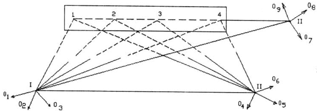
Hình 2. Quan trắc chuyển dịch ngang bằng phương pháp đo hướng
