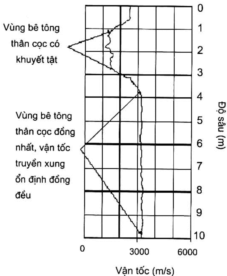
Hình C3 - Sự suy giảm của vận tốc truyền xung siêu âm trong vùng bê tông có khuyết tật.
