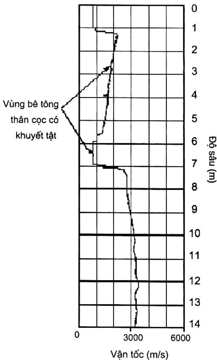
Hình B - Biểu đồ vận tốc truyền xung siêu âm.
