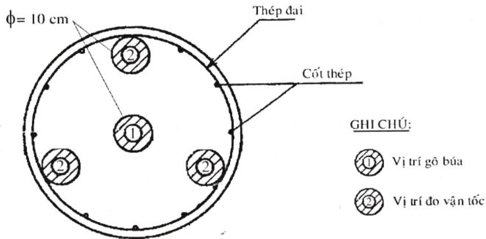
Hình 1 - Sơ đồ bố trí các điểm đo
