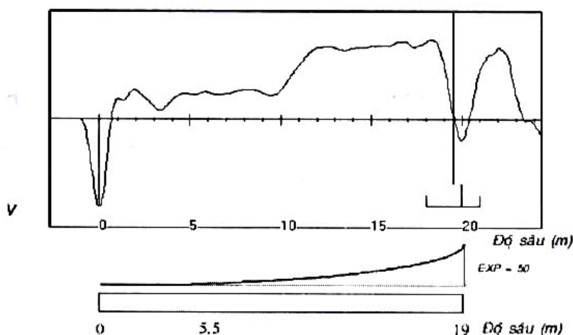
Hình 2 - Biểu đồ vận tốc
