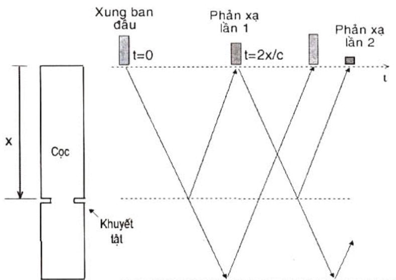
Hình A.1 - Quá trình truyền sóng trong cọc
