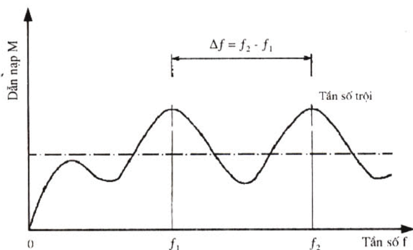
Hình 3 - Biểu đồ độ dẫn nạp của cọc
