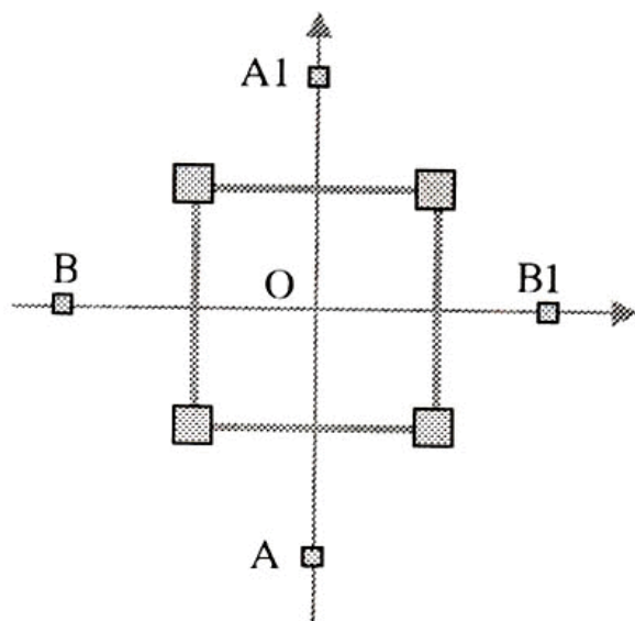
Hình 4. Sơ đồ xác định độ nghiêng của tháp truyền hình và ăng ten VTTH
