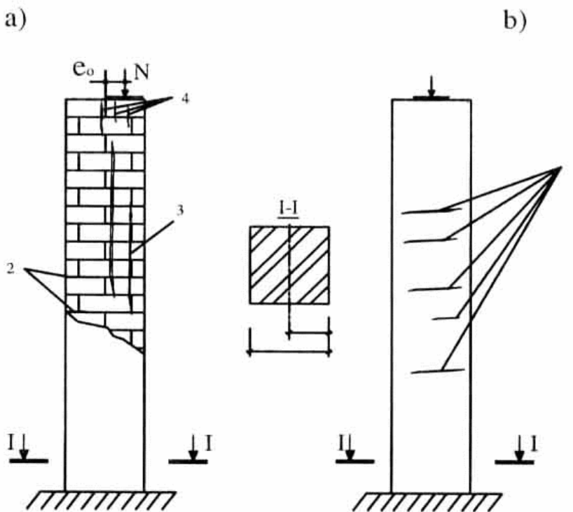
Hình C.1 - Vết nứt trong tường, trụ gạch
