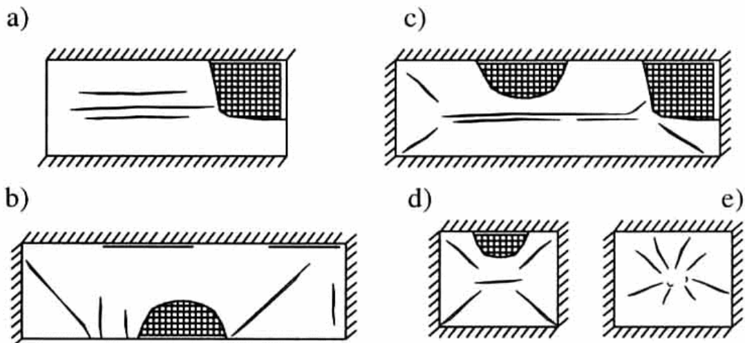
Hình B.1 - Vết nứt do tác động của lực trong bản sàn
