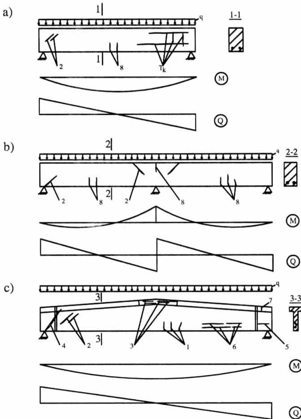
Hình B.3 - Vết nứt trong dầm
