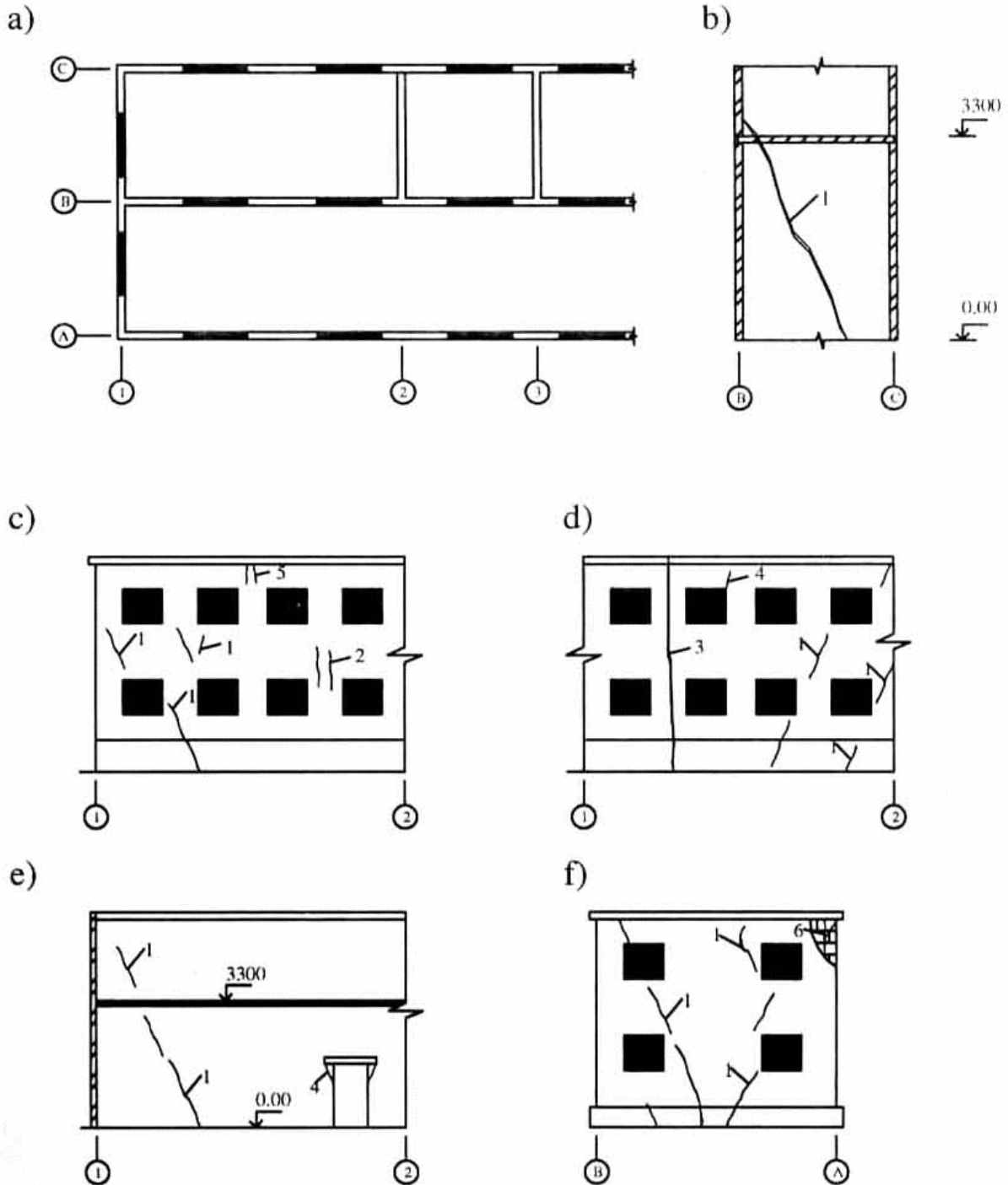
Hình C.2 - Vết nứt trong tường
