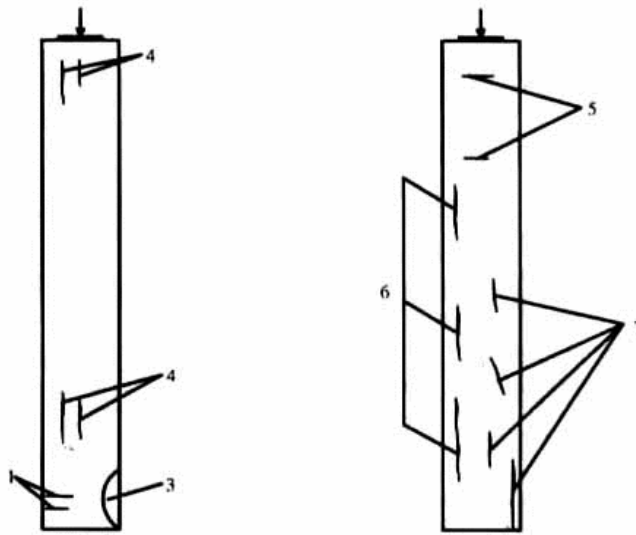
Hình B.4 - Vết nứt trong cột bê tông cốt thép
