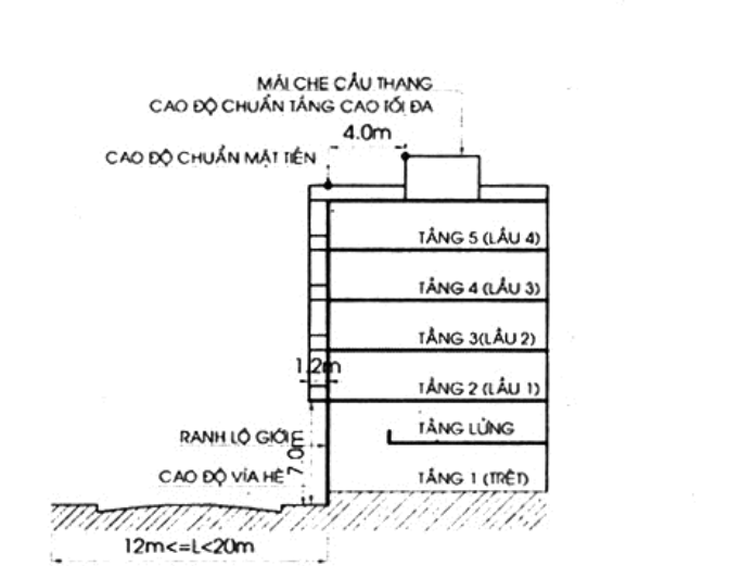
12m \leq L < 20m : ban công nhô ra tối đa 1,2m
