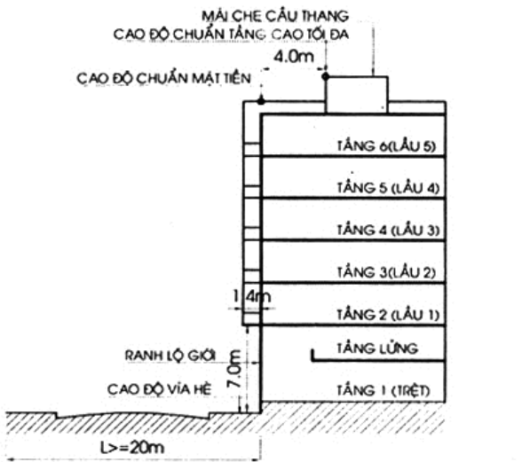
L \geq 20m : ban công nhô ra tối đa 1,4m
