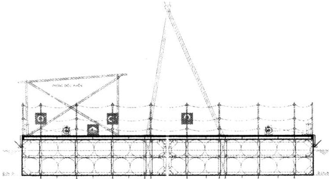
Hình 2. Sơ đồ lắp ghép giàn khoan (nhìn ngang)
