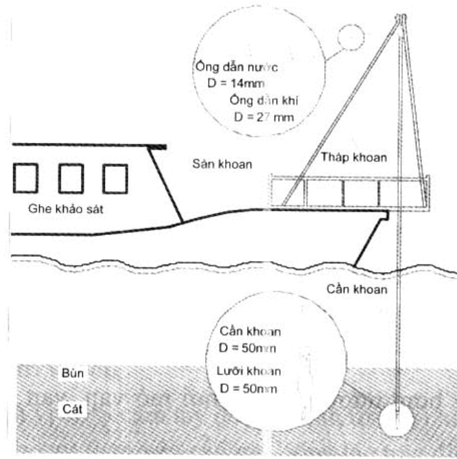
Hình 4. Nguyên lý hoạt động của phương pháp khoan thổi
