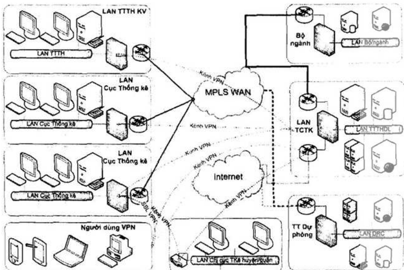
Hình 1. Sơ đồ tổng thể của mạng GSONet
