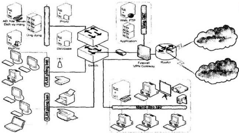
Hình 4. Sơ đồ mạng LAN tại các Trung tâm Tin học Thống kê khu vực
