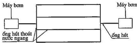
a) Sơ đồ hệ thống ống hút thoát nước ngang dạng mạng lưới.
