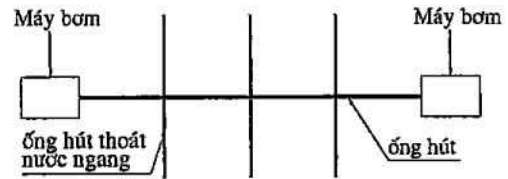
b) Sơ đồ hệ thống ống hút thoát nước ngang dạng mạng xương cá.
