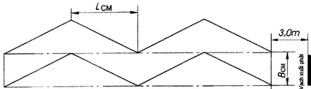
Hình bài sát hạch tiến và lùi qua hình chữ chi hạng A3, A4
