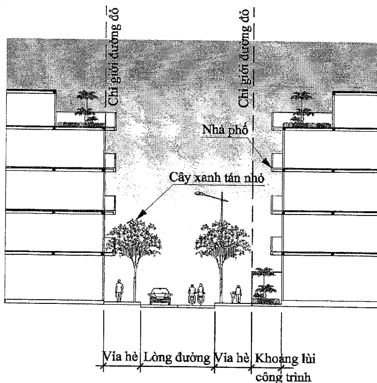
Hình 48-5 Minh họa tổ chức không gian kiến trúc, cảnh quan tuyến đường nhóm nhà
