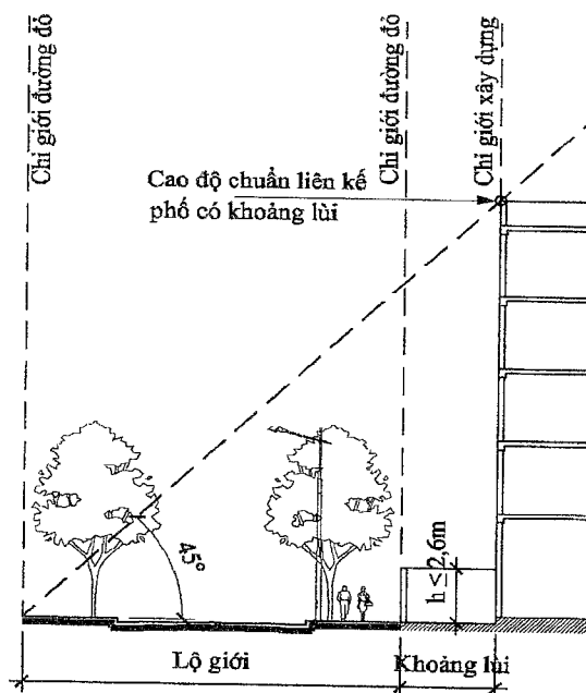
Hình 42-1 Cao độ chuẩn nhà liên kế phố có khoảng lùi
