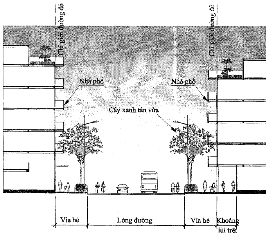
Hình 48-4 Minh họa tổ chức không gian kiến trúc, cảnh quan tuyến đường khu vực
