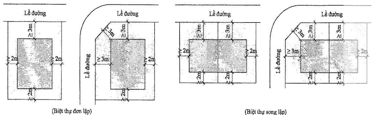
Hình 30-2 Chỉ giới xây dựng biệt thự
