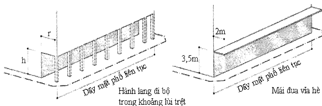
Hình 41-3 Vĩa hè - Hành lang đi bộ
