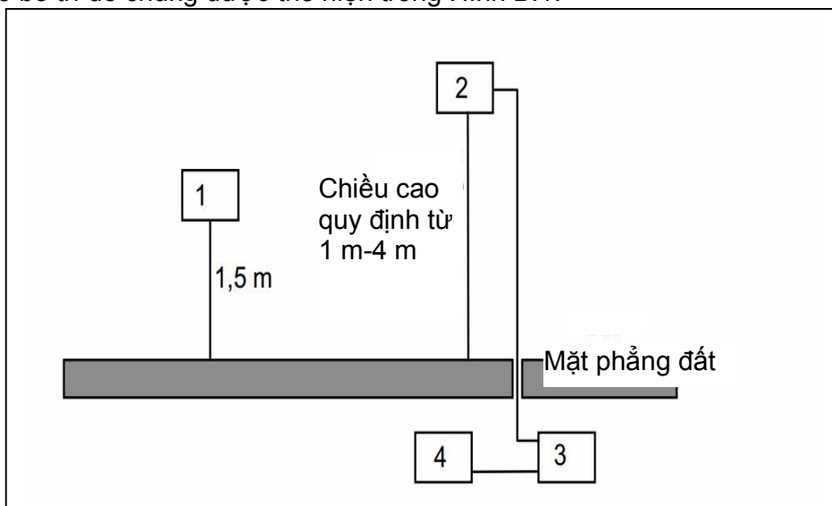
Hình B.1- Bố trí phép đo
