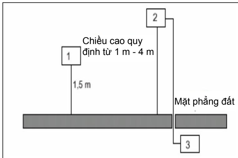
Hình C.1- Bố trí phép đo số 1
