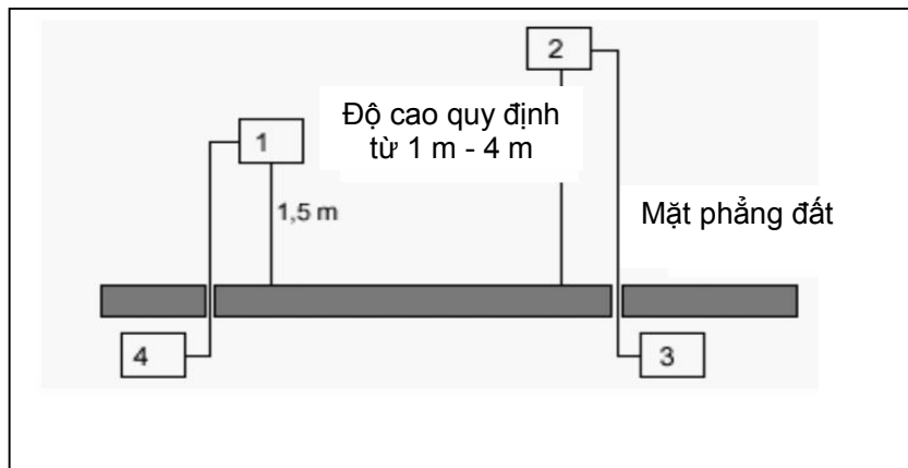
Hình C.2 - Bố trí phép đo số 2
