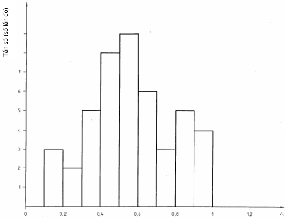
Hình E.3 Sự phân bố tần số r_N (rung động theo phương thẳng đứng)
