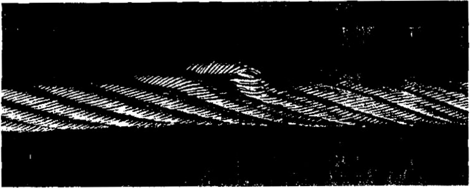
Hình B.4 – Táo cáp nhô ra hoặc bị bóp méo
