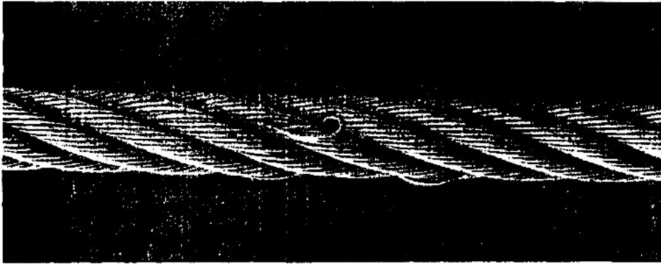
Hình B.1 – Sợi nhô ra
