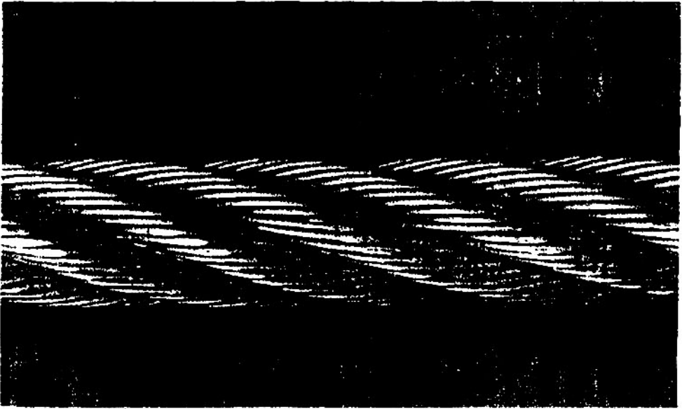
Hình B.14 – Đứt sợi vùng lõm
