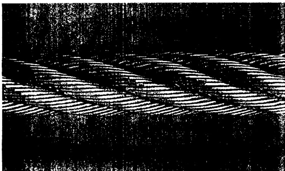
Hình B.13 – Đứt sợi vùng lỗi
