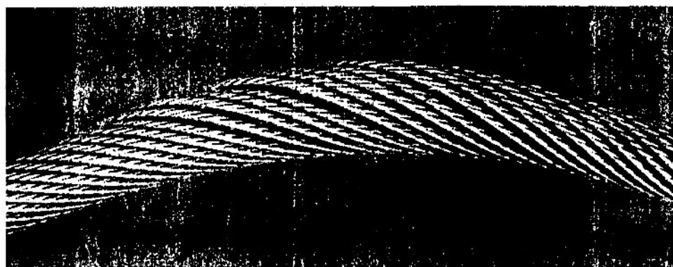
Hình B.9 – Cáp bị phồng
