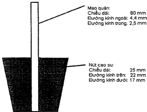
Hình 2 – Nút cao su có ống mao quản thủy tinh
