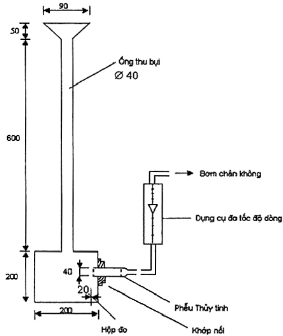
Hình 1 – Dụng cụ đo bụi
