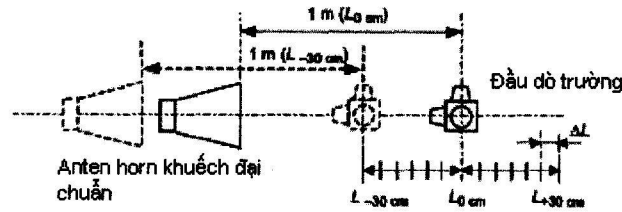
Hình I.7 - Thiết lập phép kiểm tra sự hợp lệ của buồng đo
