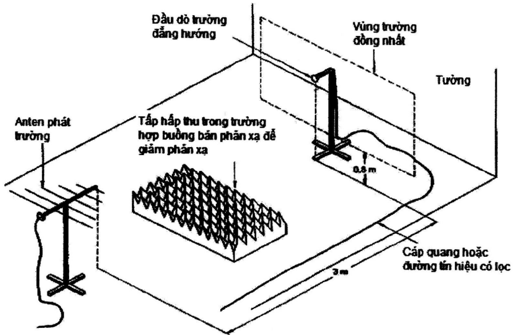
Hình 3 - Hiệu chuẩn trường
