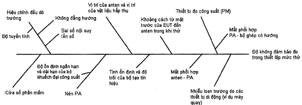
Hình J.1 - Ví dụ ảnh hưởng của việc thiết lập mức đo
