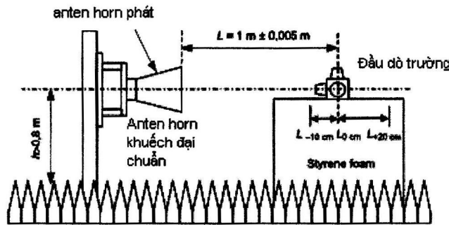
Hình I.3 - Thiết lập phép kiểm tra tính xác thực của bùồng đo
