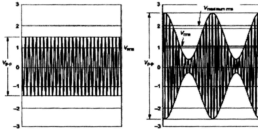
a) Tín hiệu RF chưa điều chế
