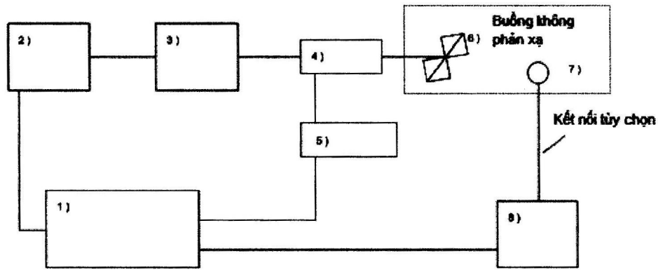
Hình 7 - Thiết lập cấu hình đo
