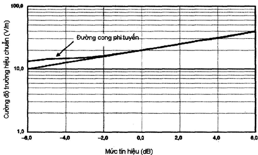
Hình 1.1 - Ví dụ về đặc tính tuyến tính của đầu dò
