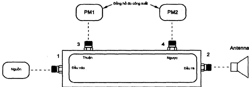
Hình 1.2 - Thiết lập phép đo công suất nguồn đến một thiết bị phát
