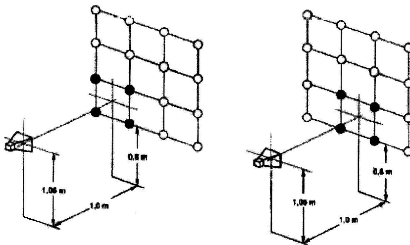
Hình H.2 - Ví dụ về chiều rọi các cửa sổ liền kề
