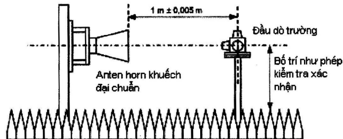
Hình I.9 - Bố trí hiệu chuẩn đầu dò trường
