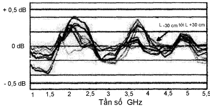
Hình I.8 - Ví dụ về dữ liệu đánh giá buồng đo của phương pháp thay thế.
