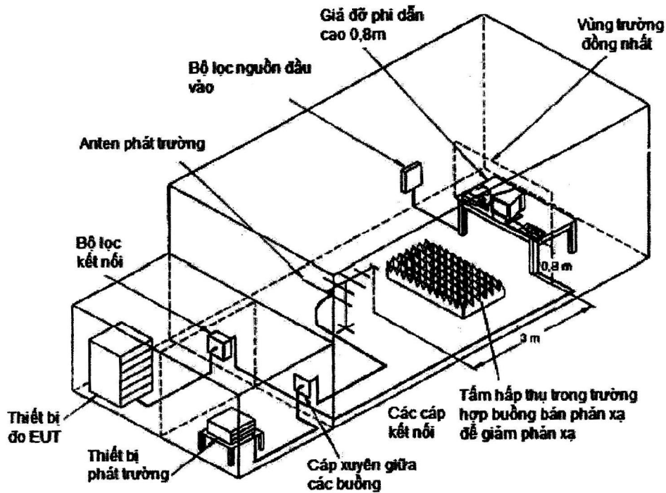
Hình 2 - Ví dụ về phương tiện thử
