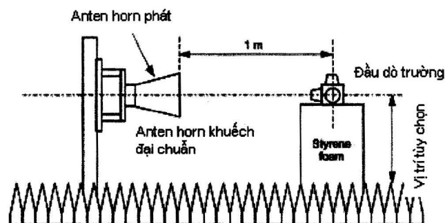
Hình 1.6 - Ví dụ bố trí phép thử cho anten và đầu dò.
