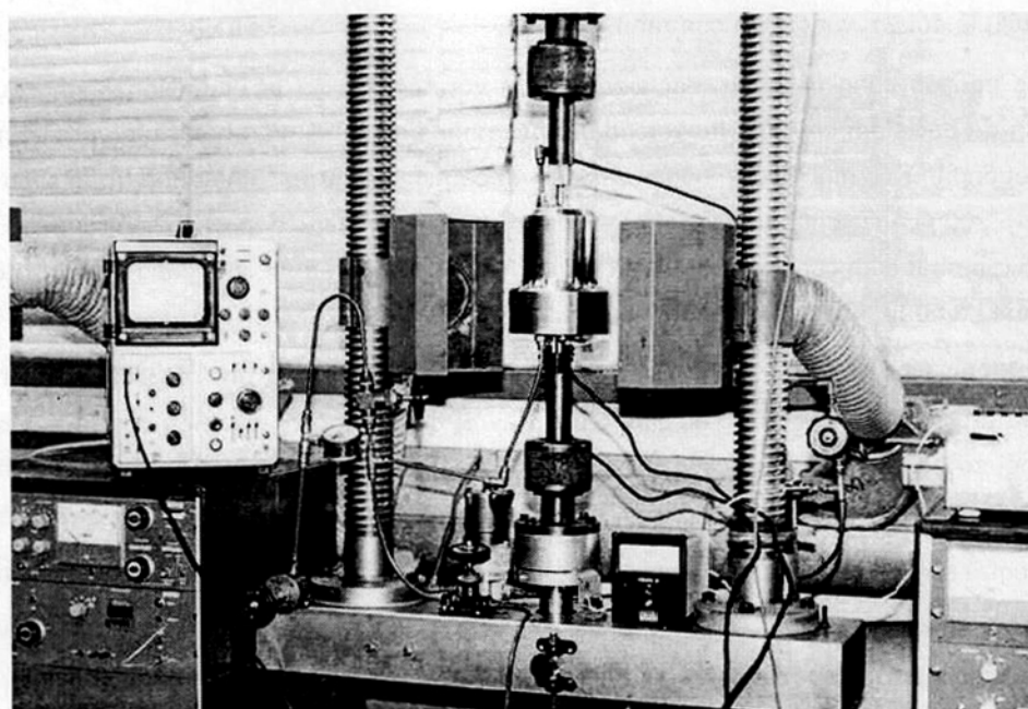
Hình 7 – Máy thử thủy lực secvo
