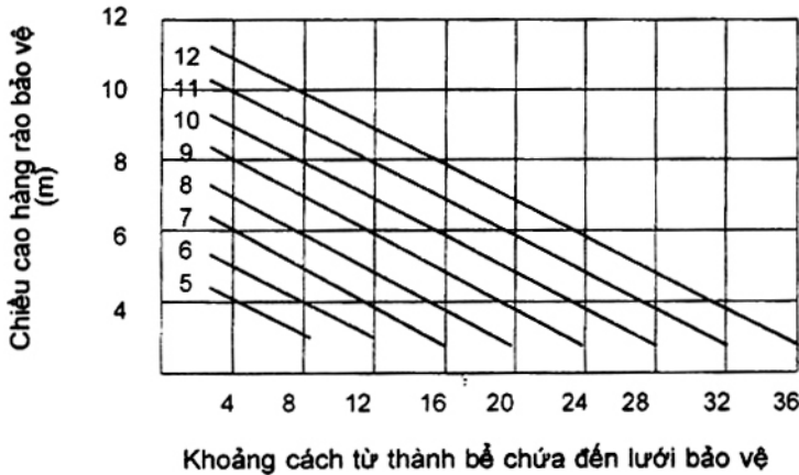
Hình 1 - Đồ thị xác định chiều cao hàng rào bảo vệ
