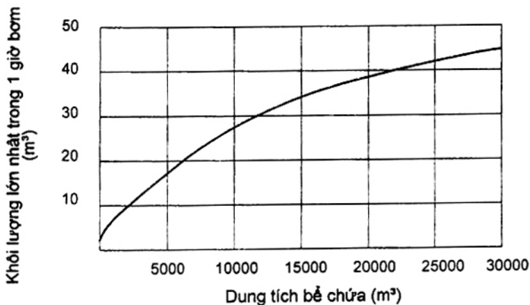
Hình 2 - Đồ thị xác định năng suất máy bơm
