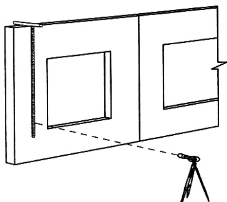
Hình 48- Đo cao độ cầu kiện bằng cách treo mìa thủy chuẩn lên đó
