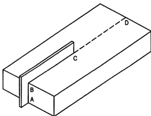
Hình 13- Phương pháp sử dụng khi không có sai lệch đường thẳng
