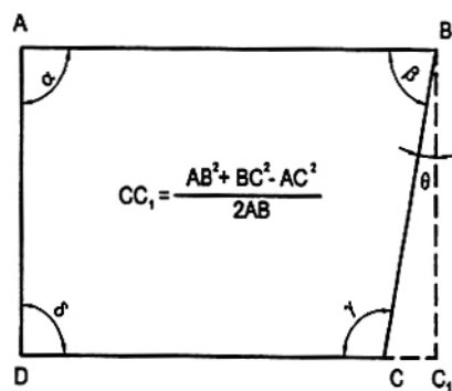
Hình 14- Xác định các khoảng cách AB, BC, AC
