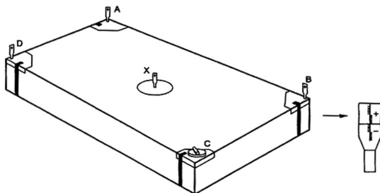
Hình 27- Ví dụ đo độ phẳng với mặt phẳng chuẩn đi qua ba điểm góc
