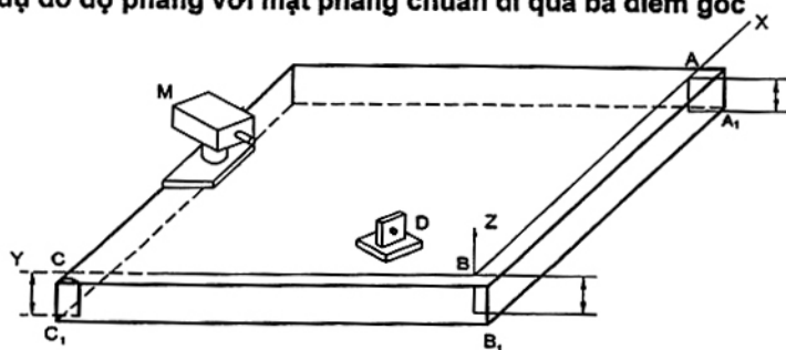
Hình 28- Ví dụ đo độ phẳng bằng thiết bị tiêu cực ngăn không bù trừ
