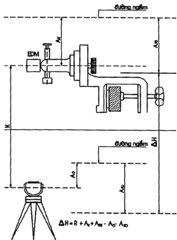
Hình 74- Mô tả phương pháp đo bằng máy EDM.
