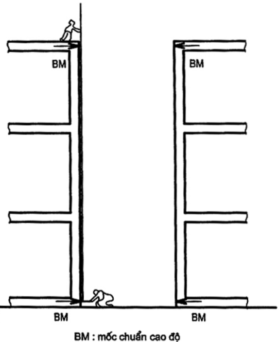
Hình 72- Đo chiều cao khoảng trống hồ thang máy
