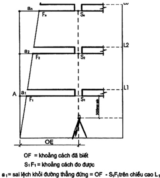
Hình 53- Xác định độ sai lệch khỏi đường thẳng đứng bằng máy đo quang học
