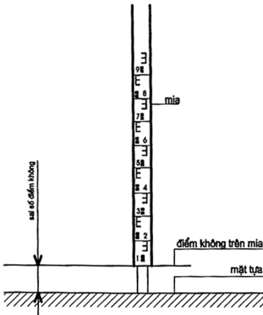
Hình 71- Trường hợp có sai số điểm không
