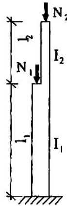
Hình D.1 – Sơ đồ cột một bậc
