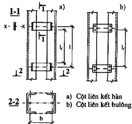
Hình 5 – Cột tổ hợp bằng bản giằng
