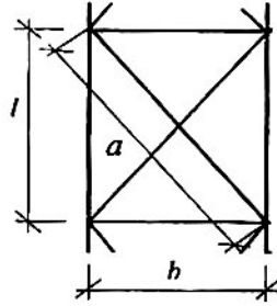
Hình 6 – Sơ đồ thanh giằng chữ thập
