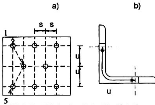
Hình 1 – Cách xác định diện tích thực
