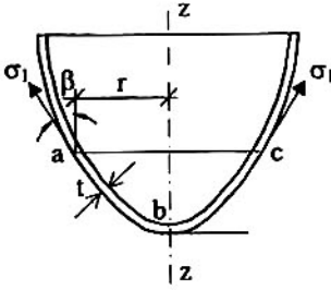
Hình 15 – Sơ đồ vỏ tròn xoay
