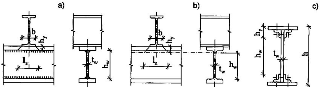
a) Dầm hàn; b) Dầm thép cán; c) Dầm bulông (đỉnh tán)
