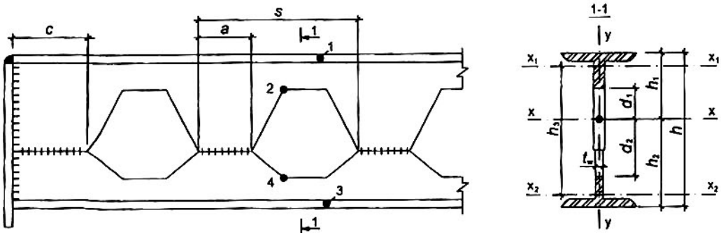
Hình 20 – Sơ đồ một đoạn dầm có lỗ
