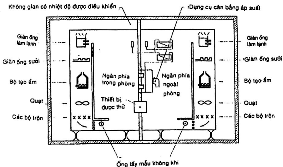
Hình B.5 – Nhiệt lượng kế kiểu buồng điển hình cân bằng môi trường xung quanh
