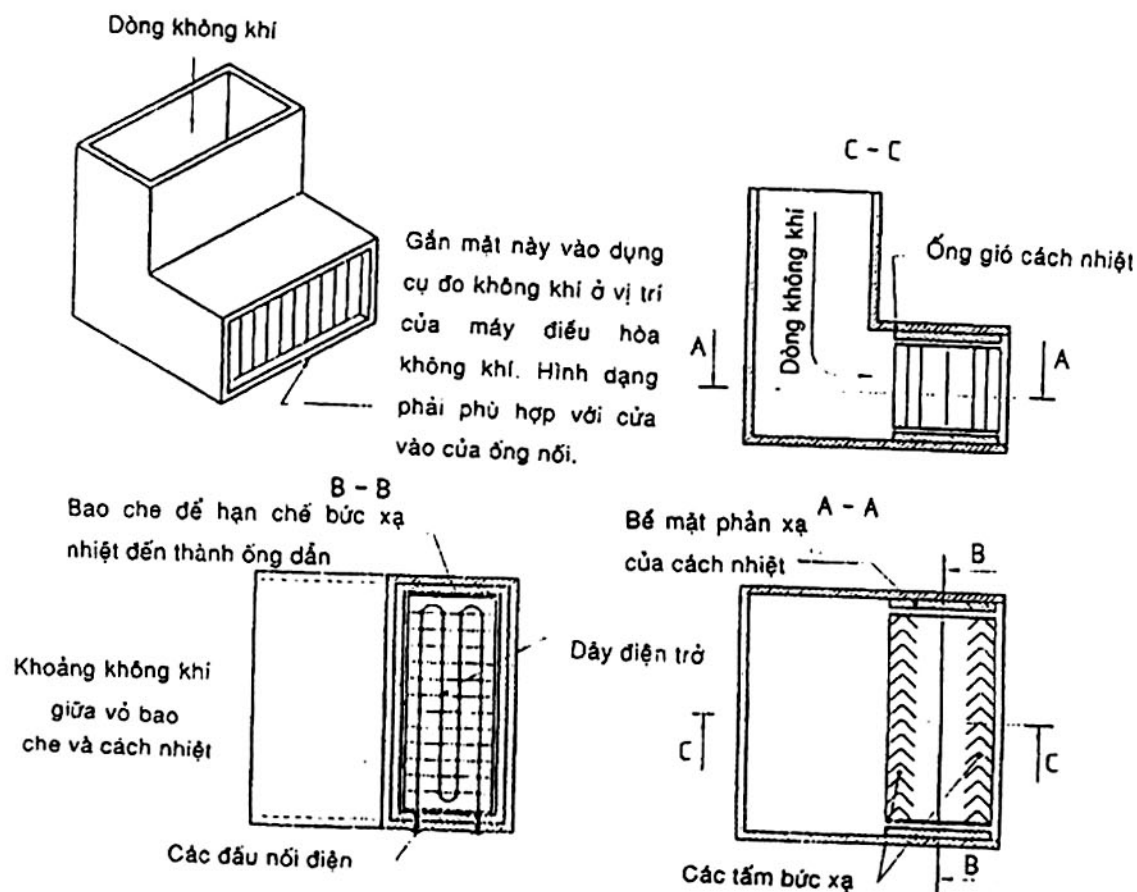
Hình C.1 – Trang bị thử tiêu chuẩn
