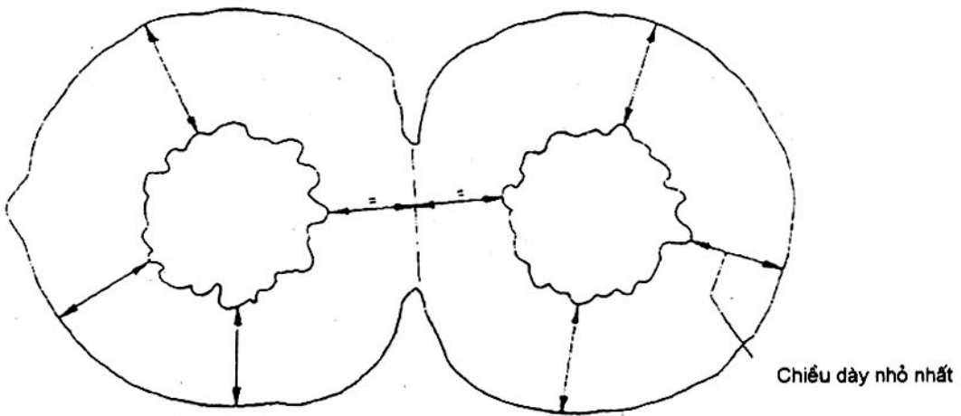
Hình 5 - Đo chiều dày cách điện (biên dạng mặt ngoài không nhẵn)
