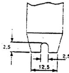
Hình 14 – Đầu chày đột dập có rãnh
