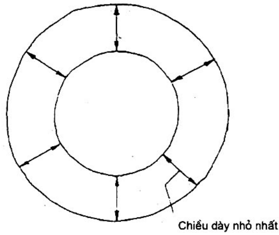
Hình 1 – Đo chiều dày cách điện hoặc vỏ bọc (biên dạng bên trong tròn)
