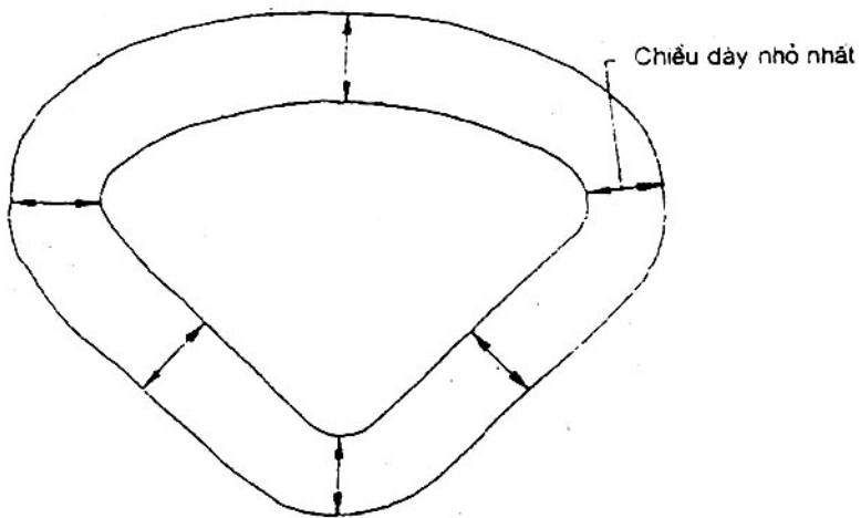
Hình 2 – Đo chiều dày cách điện (ruột dẫn có hình chữ nhật)
