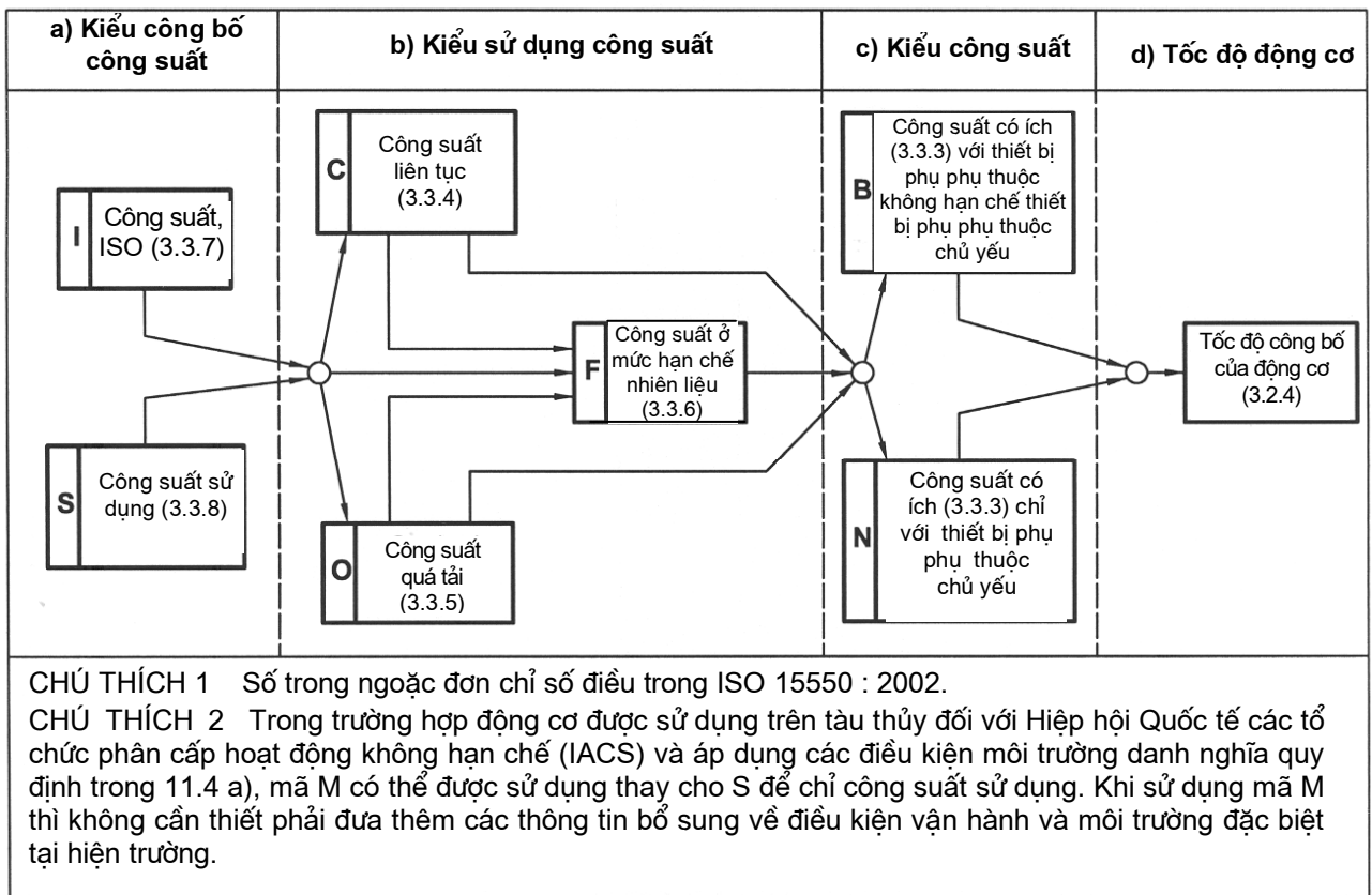
Hình 2 - Sơ đồ trình tự các chữ được sử dụng để mã hóa việc công bố công suất
