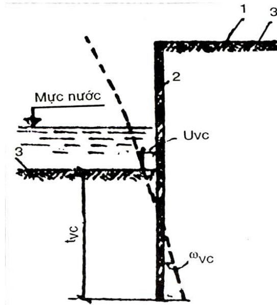
Hình 8: Sơ đồ tính nền các kết cấu ván cừ (tường) không néo theo biến dạng 1. bề mặt khu đất; 2. ván cừ, 3. mặt đáy thiết kế
