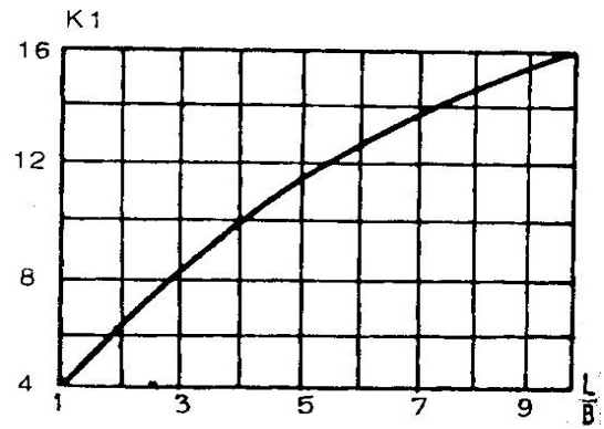
Hình 4- Các biểu đồ để xác định các hệ số k_1 và k_2
