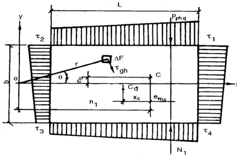
Hình 1. Sơ đồ tính toán ổn định công trình (đặt không sâu) khi trượt phẳng có quay trong mặt bằng
