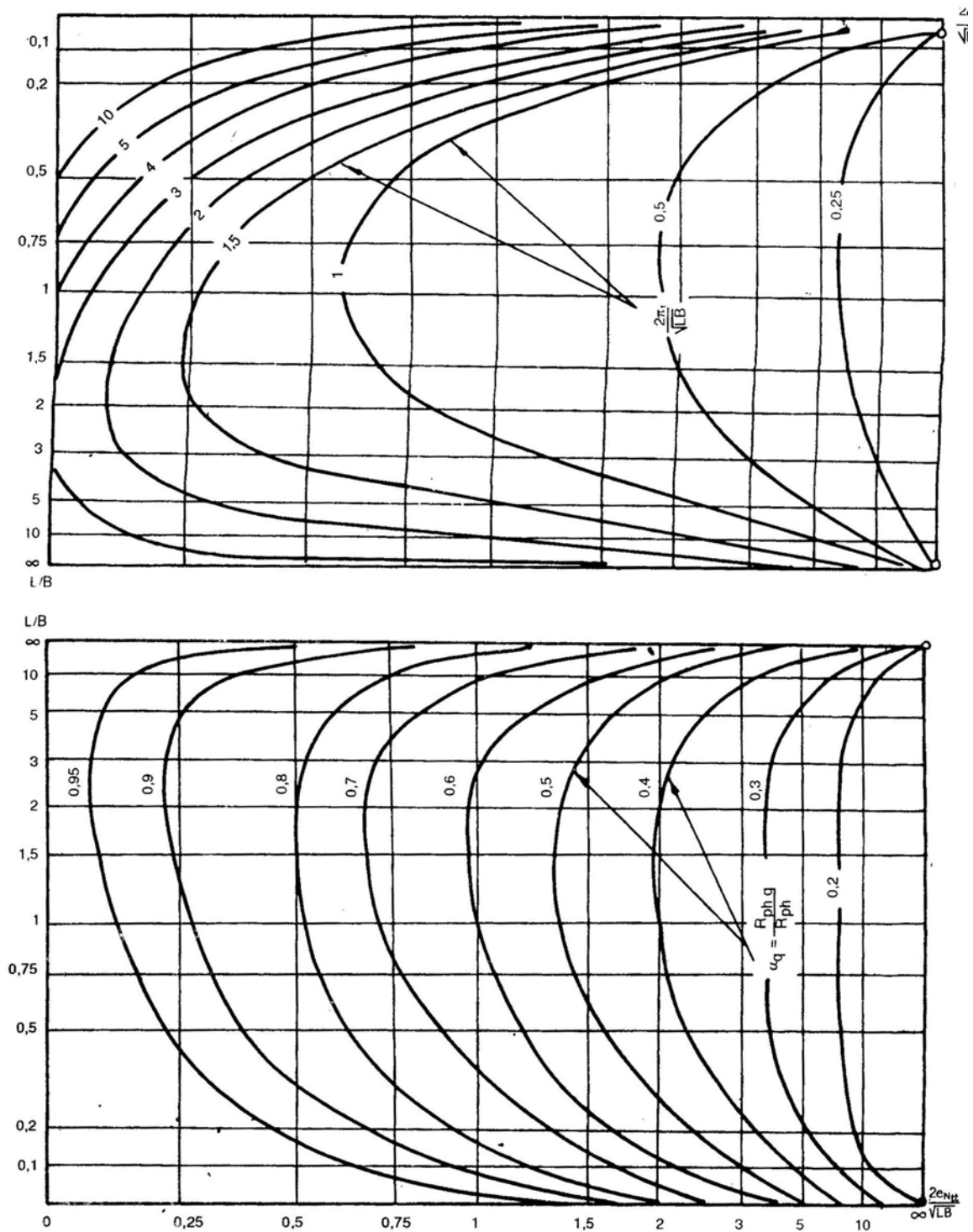
Hình 2. Các biểu đồ để xác định hệ số \alpha_q và tọa độ tâm quay n_1 và E_{bh1} - được ký hiệu như trong điều 3.4.5 của tiêu chuẩn này ;
