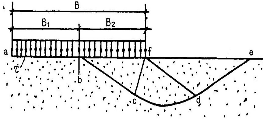
Hình 1 Sơ đồ tính sức chịu tải của nền và sự ổn định của công trình khi trượt hỗn hợp ab - Phần trượt phẳng; bf - Phần trượt có ép trôi; bedef – vùng ép trôi
