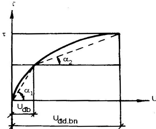
Hình 7 : Biểu đồ tính toán chuyển vị ngang giới hạn của công trình
