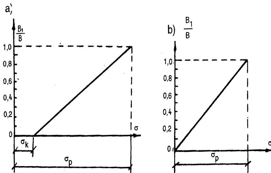
Hình 2. Các đồ thị để xác định chiều rộng của phần đáy móng công trình B_1 , tại đó xảy ra trượt có ép trời đất nền.
