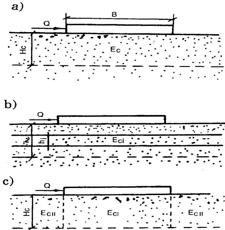
Hình 6: Các sơ đồ để xác định chuyển vị ngang của công trình
