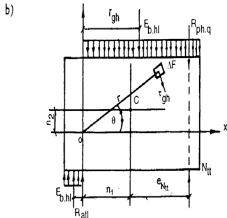
Hình 3. Các sơ đồ để tính toán ổn định công trình đặt sâu khi trượt phẳng có quay trong mặt bằng.
