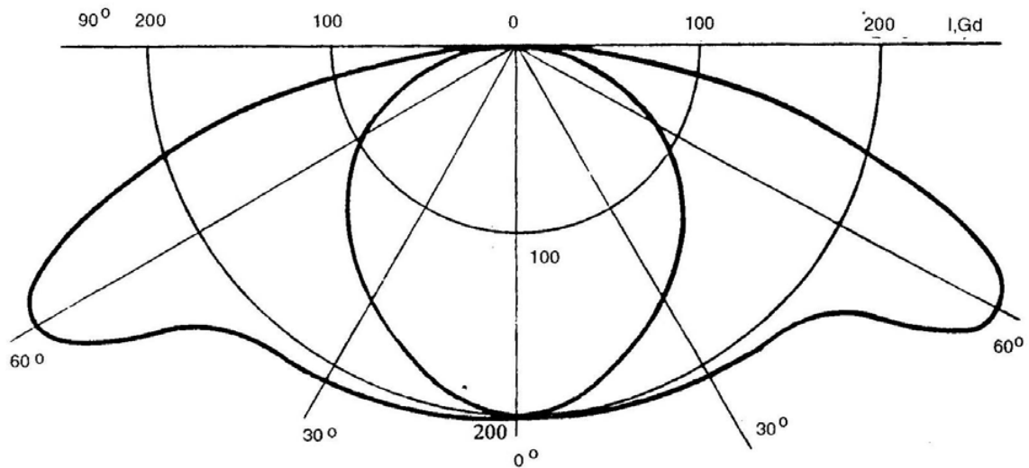
Hình 1 : Đường cong phân bố cường độ sáng
