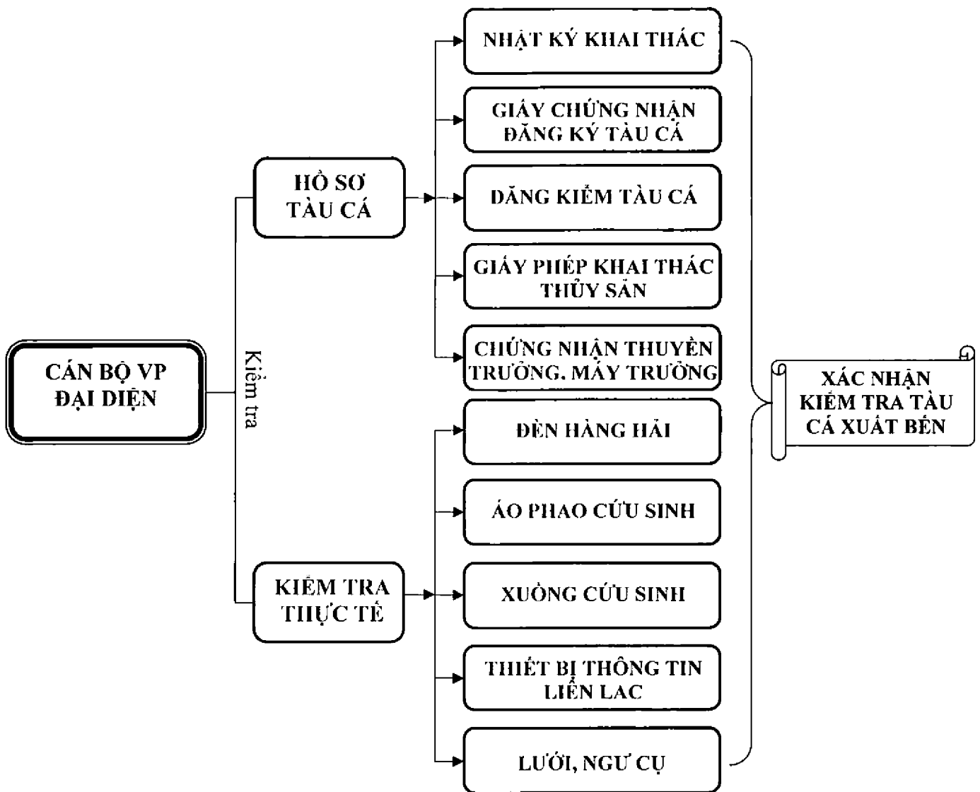
Phụ lục 2: Sơ đồ minh họa quy trình kiểm tra trước khi tàu rời cảng
