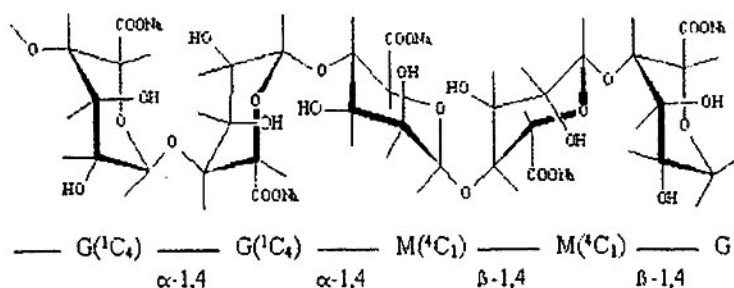
Hình 1 – Công thức cấu tạo của natri alginat
