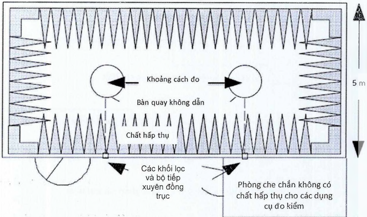
Hình A.4 - Ví dụ về cấu trúc của phòng đo không dội được che chắn
