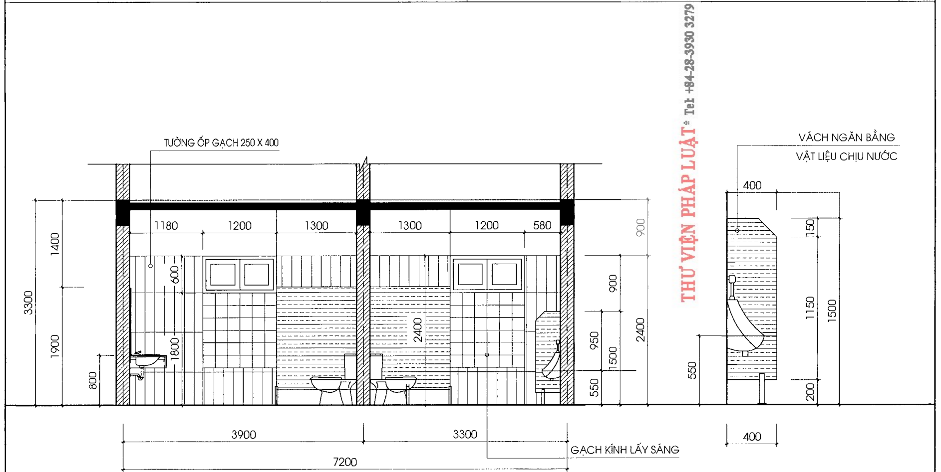
MẶT CẮT 1-1
