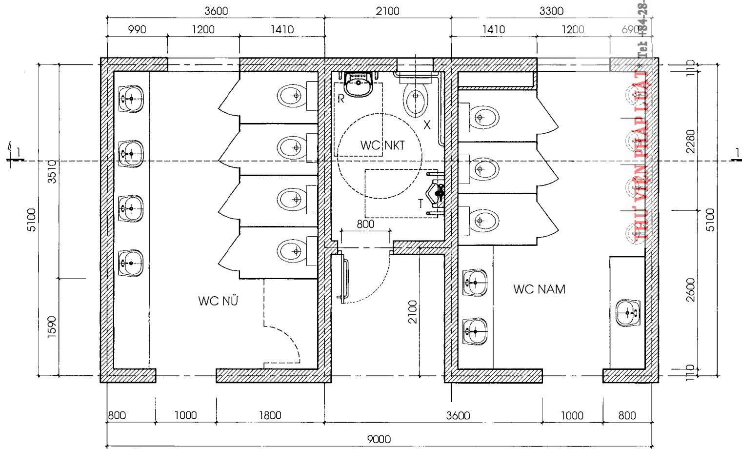
MẶT BẰNG
