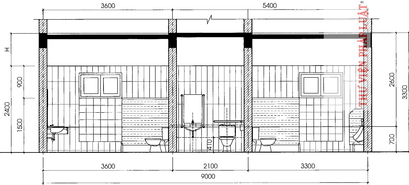
MẶT CẮT 1-1
