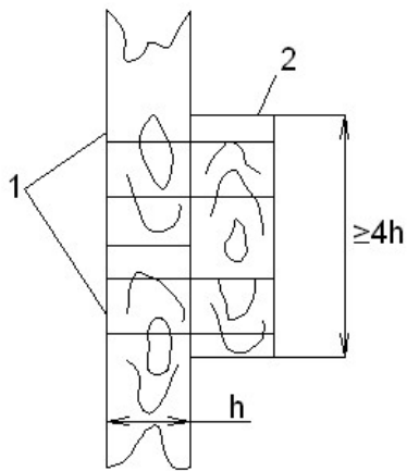
Hình 4. Mỗi nối tấp sườn đơn
