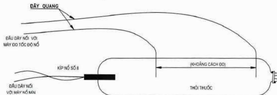
Hình 1 - Sơ đồ chuẩn bị mẫu và cách đấu dây với mẫu thuốc nỏ
